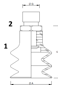
Vacuum Cup with 3 bellows (complete) Vakuumsauger mit 3 kanten (komplett) Ventosa con 3 soffiatti (completa) Ventouse avec 3 souffletts (complet) Ventosa de 3 fuelles (completa)
