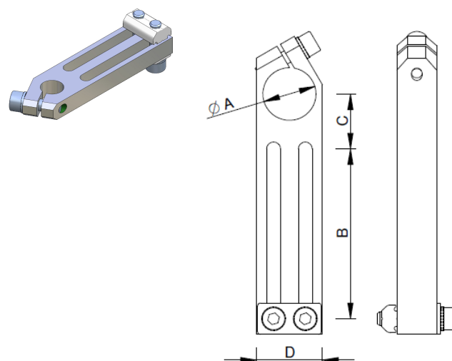
Long Angle Clamp Heavy Duty - Klemmstück Verstellbar und Verstärkt Staffa Rinforzata - Bride Robuste - Conexión Perfil
