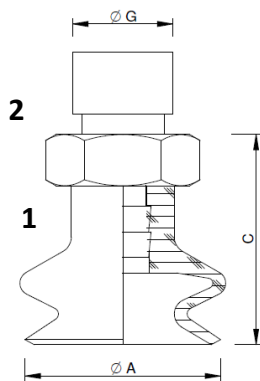
Vacuum Cup with 2 bellows (complete) Vakuumsauger mit 2 kanten (komplett) Ventosa con 2 soffiatti (completa) Ventouse avec 2 souffletts (complet) Ventosa de 2 fuelles (completa)
