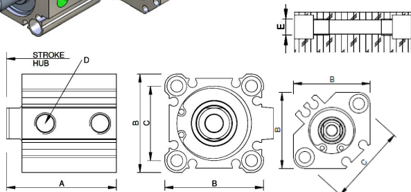
Compact Cylinder - Kompaktzylinder - Cilindro compatto Vérin Pneumatique - Cilindro Compacto
