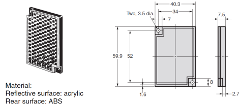
Reflector (order separately) - Rückstrahler Catarifrangente per sensori - Réflecteur - Reflector para sensor
