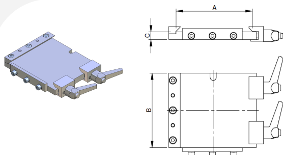
Quick changer (Robot side) - Schnellwerkzeugwechsler (Roboterseite) Cambia utensile (Lato robot) - Changeur d'outils rapide (Côté robot) Cambio rápido (Lado robot)
