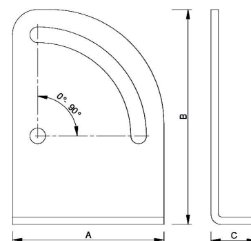
Swivel Bracket MR - Schwenkbock MR - Morsetto per attuatore MR
