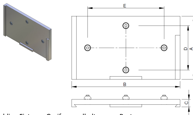
Holding Fixture - Greiferwandhalterung - Porta mano Équipement tenant - Accesorio de Tenencia
