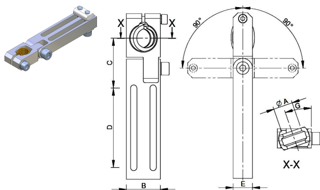
Long Angle Clamp Swivel Head and Ball Joint Winkelklemmstück Gelenkig mit Kugelgelenk Staffa Snodata con Sfera - Bride Perforeé Angulaire Sphériques Pieza de apriete en escuadra con Articulación y Esfera
