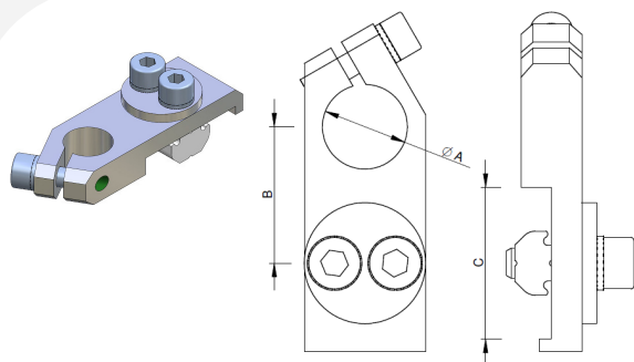
Adjustable Clamp - Klemmstück Drehbar - Staffa Angolare Bride de Fixation - Pieza de Apriete Angular
