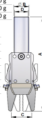
CA.GTS.1003.1415/145N CA.GTS.1004.1415/145N
