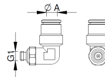
Orienting elbow male adapter (parallel) - Steckverschraubung L-Form Raccordo gomito - Équerre orientable mâle - Empalme en codo
