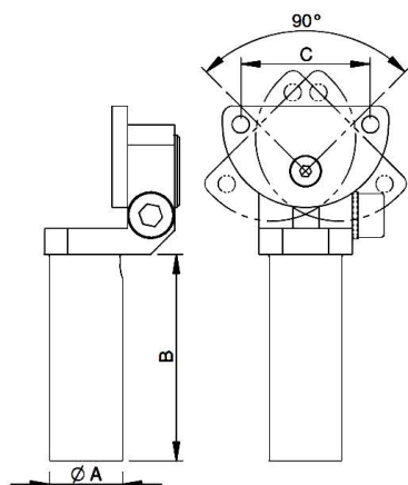
Adapter for Part Control - Adapter für Teilekontrolle Staffa Snodata per Sensore - Bras de Prise Estribo para Sensor
