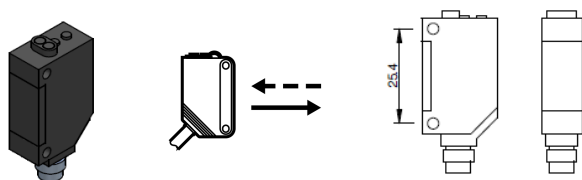
Distance-settable (Laser) - Hinter-/Vordergrundausbldung (Laser) Fotosens. sopp. di sfondo regolabile - Distance réglable Sensor fotoeléctrico tipo distance - settable
