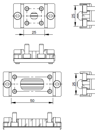
Profile End Connector 25 - Stoßverbinder 25 Connessione Terminale per Profilo 25 Fixation Verticales pour Profilés 25 Conexión Terminal para Perfiles 25
