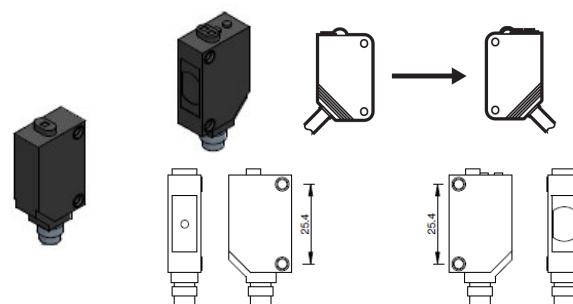
Through-beam laser 1 mm - Einweglichtschranke Laser 1 mm Fotosens. spot 1 mm emett./ricev - Barrage Sensor fotoeléctrico tipo through-beam
