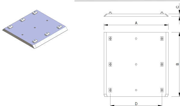
Quick changer (Gripper side) - Schnellwerkzeugwechsler (Greiferseite) Cambia utensile (Lato mano) - Cambio rápido (Lado pinza) Changeur d'outils rapide (Côté main de préhension)
