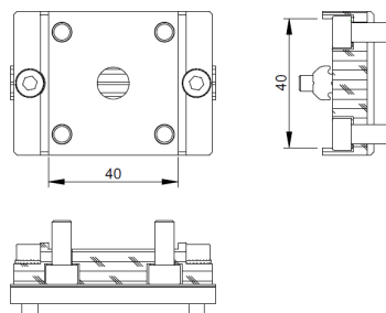
Profile End Connector 40 - Stoßverbinder 40 Connessione Terminale per Profilo 40 Fixation Verticales pour Profilés 40 Conexión Terminal para Perfiles 40
