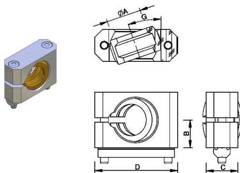
Cross Connector Round With Ball Joint Kreuzklemmstück Rund mit Kugelgelenk Connessione Tubo con Sfera Bride Ronde pour Fixation en Croix avec Boule Pieza de Apriete en Cruz con Esfera
