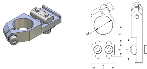
Adjustable Clamp - Winkelklemmstück - Staffa Angolare Bride de Fixation - Pieza de Apriete Angular
