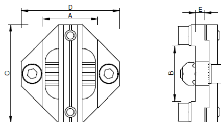
Cross Joint Connector - Profilverbinder - Connessione a Croce Brides pour Fixation en Croix - Placa en Cruz para Perfiles
