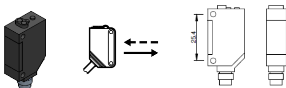
Laser Thin beam type (1 mm) reflective model Laser Reflexionslichttaster mit engem Strahlkegel (1 mm) Fotosens. tast. diretto fascio (1 mm) Détection et positionnement précis Sensor fotoeléctrico tipo thin beam (1 mm) modelo reflectivo
