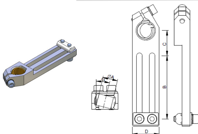
Long Angle Clamp with Ball joint Klemmstück Verstellbar mit Kugelgelenk - Staffa con Sfera Bride de Fixation Universel avec Boule Pieza de Apriete en Escuadra con Esfera
