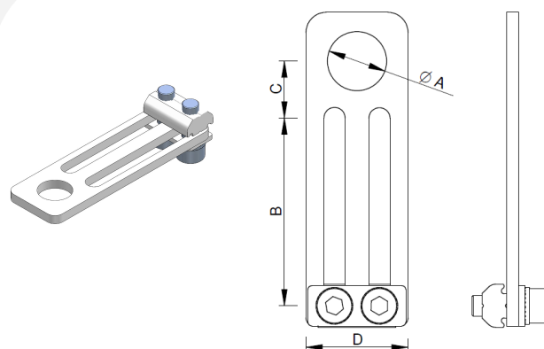
Mounting Bracket - Klemmstück Verstellbar - Staffa Passaparete Bride de Fixage - Conexión Perfil - Pistón Pequeño
