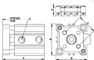
Compact Cylinder/Guide Rod Type Kompaktzylinder mit Führungsstangen Cilindro Antirotazionale - Vérin Pneumatique Cilindro Compacto Antitorsión
